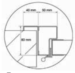
Присоединительные размеры
