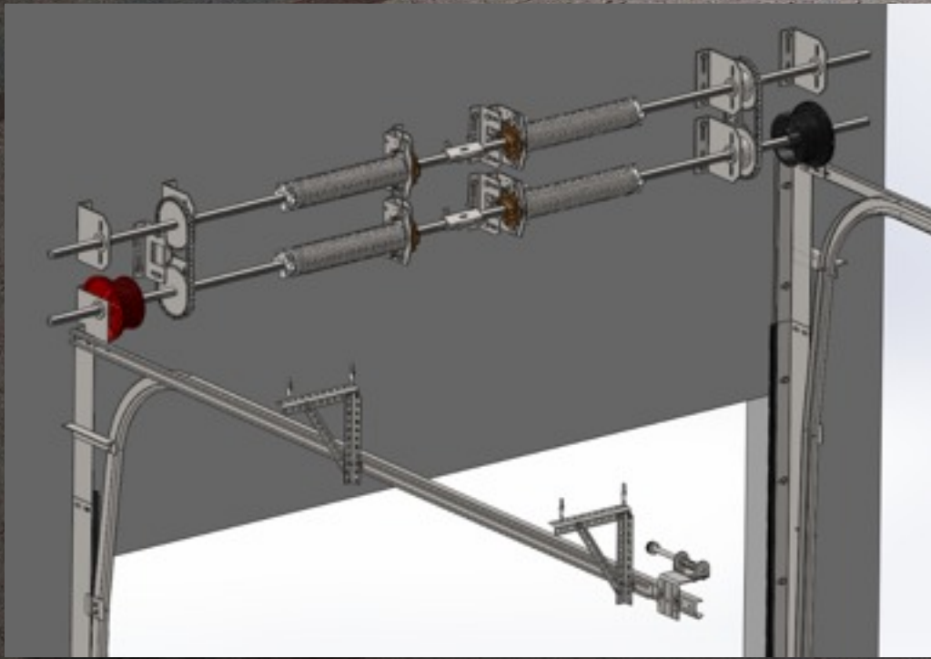
синхронизация с помощью цепи
