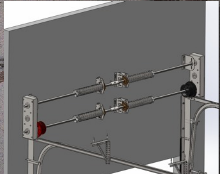
синхронизация с помощью редуктора
